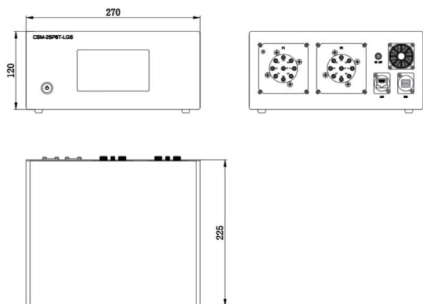
外形图
