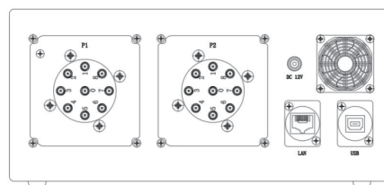
外形图
